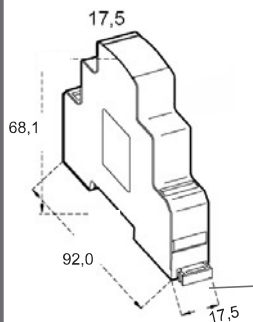
GEHÄUSE / CASE 1M
