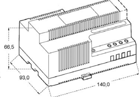
GEHÄUSE / CASE 8M
