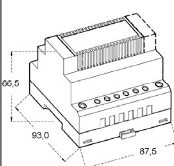
GEHÄUSE / CASE 5M
