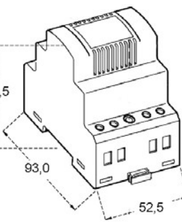
GEHÄUSE / CASE 3M
