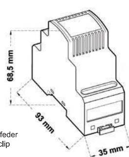
GEHÄUSE / CASE 2M
