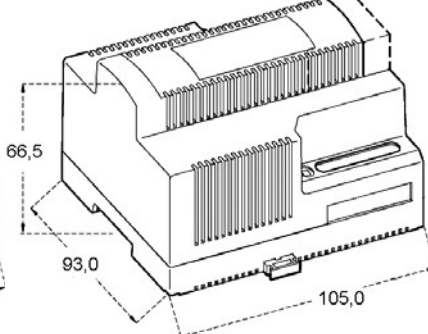
GEHÄUSE / CASE 6M
