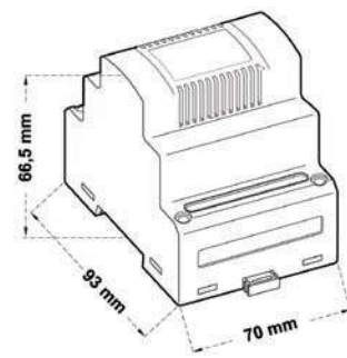
GEHÄUSE / CASE 4M
