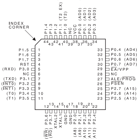
PQFP/TQFP
